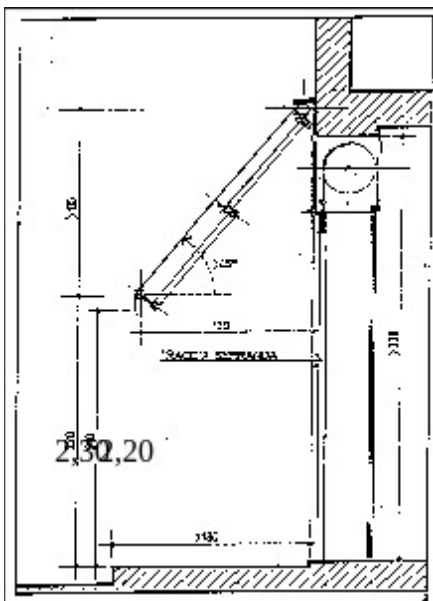
Fig. 2. Vale quanto detto nell'esempio precedente. In questo caso può l'altezza del vano vetrina = 330 cm. permettere il rispetto ottimale della distanza di 20 cm. attorno al profilo della bucatura.
