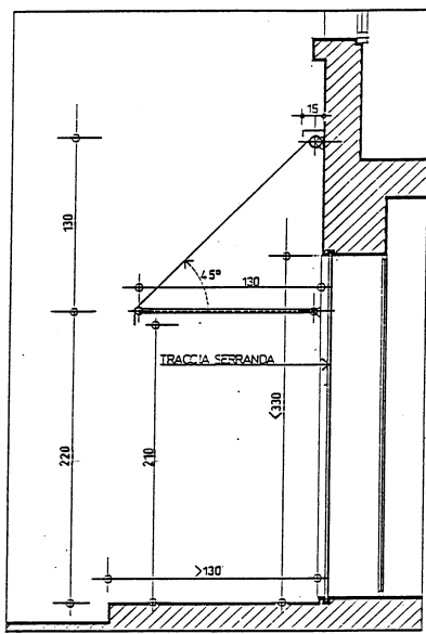
Fig. 1. Vano vetrina con h > 330 cm. È consentito l'uso della tenda a meccanica tradizionale con rullo raccoglitore a un'altezza sufficiente per il braccio estensore lungo 130 cm con fulcro alto 230 cm. da terra.
