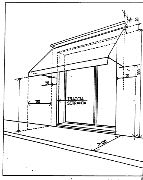
Fig. 3. Qualora il vano vetrina abbia h > 330 cm., il montaggio di un braccio estensore a tre cerniere, consentendo un'inclinazione della tenda > 45^\circ , permette che si rispetti l'altezza da terra di 220 cm. e l'aggetto di 130 cm
