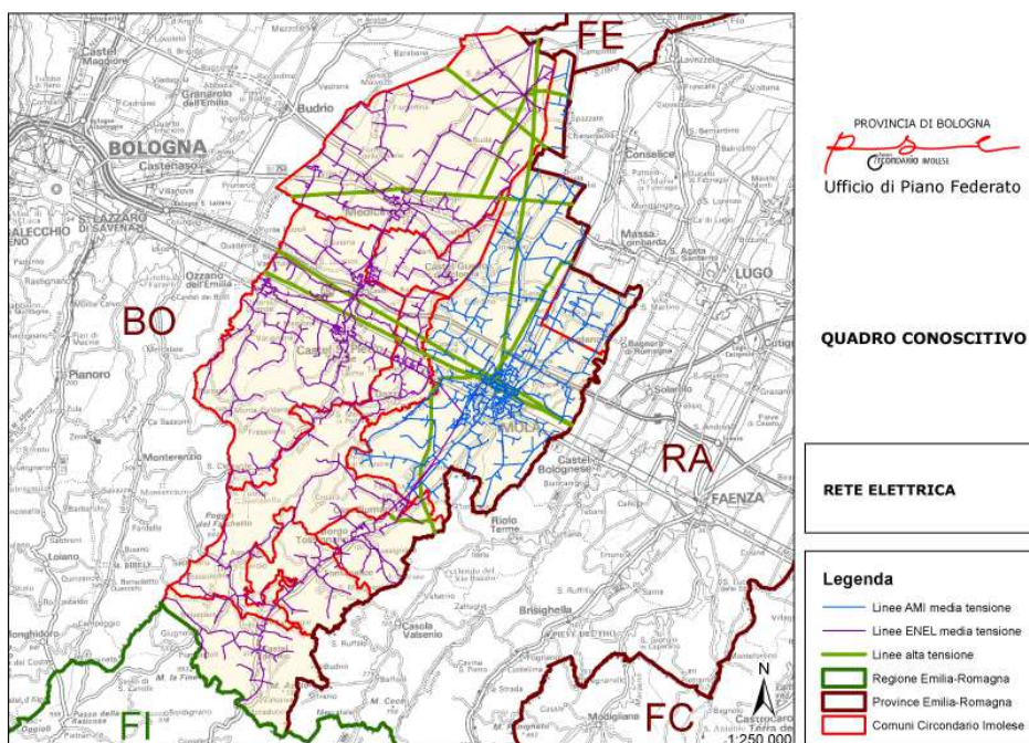
Tav. 7.- RETE ELETTRICA.
