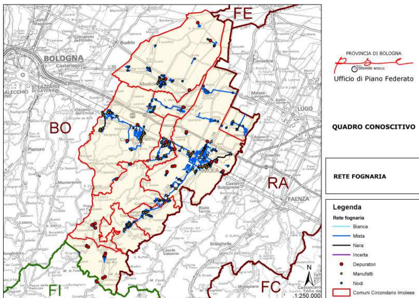
Tav. 8. - RETE FOGNARIA.
